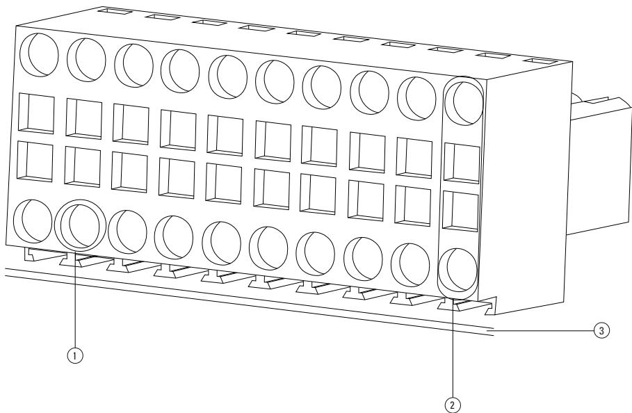
Figure 16. Alignement correct du connecteur homologue
